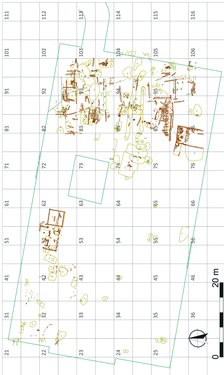
Ryc. 4. Wrocław, pl. Nowy Targ. Plan wykopu na poziomie II fazy osadniczej (oprac. M. Mackiewicz)
